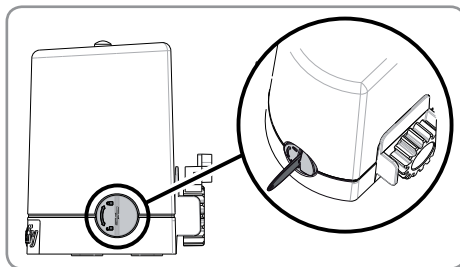
Привод разблокирован
